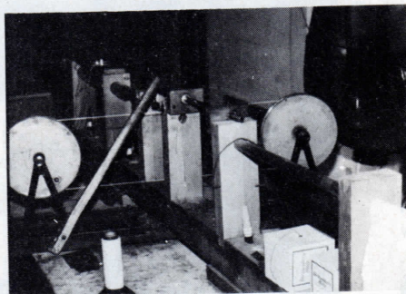
Weirs egen konstruktion. En maskin som samtidigt lindar ihop bamburibborna från motsatta håll i samband med limningen.
